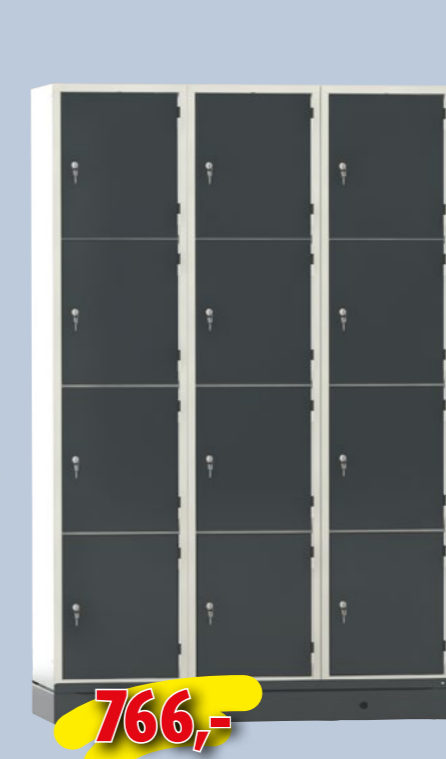
Universal-Wertfachschränk 1850 x 400/800/1200 x 500 mm H x B x T, mit 4/8/12 Abteilen. Innenmaße: 445 x 370 x 480 mm H x B x T, lichter Durchgang 420 x 330 H x B. Rückwand gelocht zur Belüftung. Türen (rechts angeschlagen) durch Zylinderschloss abschließbar. Pro Zylinderschloss 2 Schlüssel.
